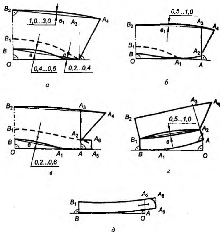
Расми 6.10. Кашидани нақшаи созаи гиребонҳо барои писарчаҳо
