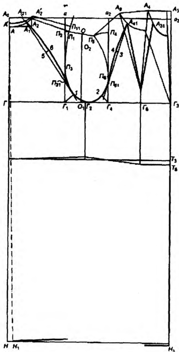
Расми 3.34. Нақшаи либос бо остини реглан
