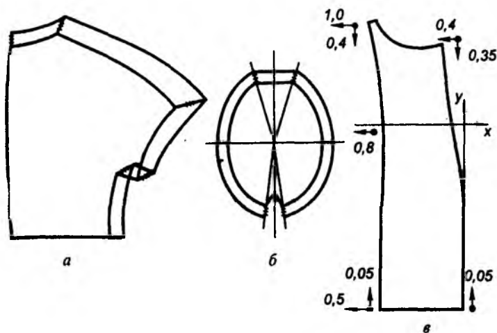
Расми 11.1. Дараҷабандии қолибҳо
