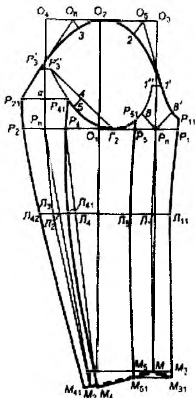
Расми 3.23. Нақшаи остини дучоқро бо чокҳои пешу оринҷӣ.
