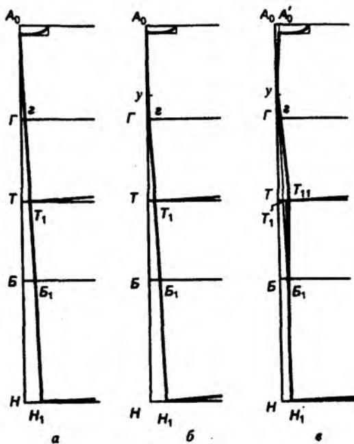
Расми 5.6. Кашидани хати мобайни пуштак дар либос барои духтарчаҳо
