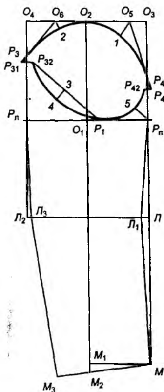
расми 6.7. Кашидани нақшаи асоси остини даврадӯзӣ
