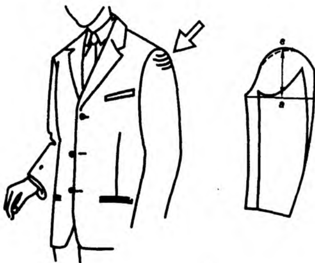
расми 13.10. Чинҳом арзӣ дар қисми болои сари остин
