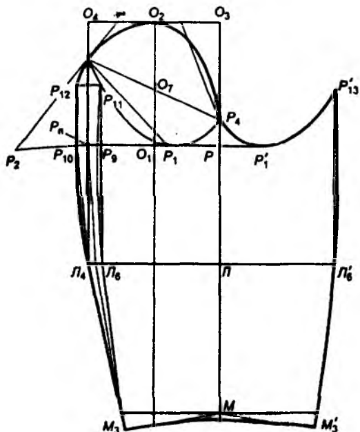
Расми 4.9. Кашидани нақшаи созаи остини якчока (бо чоки оринҷӣ)
