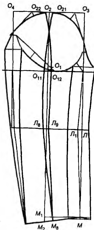
Расми 6.9. Кашидани нақшаи сози остини сечока
