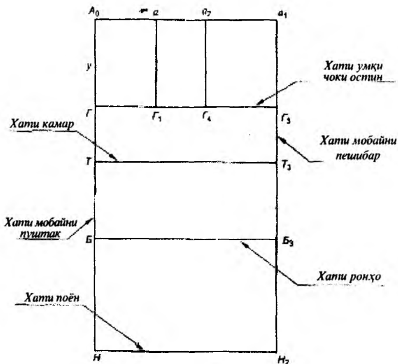
Расми 3.11. Нақшаи тарҳи асосӣ барои сохтани асоси либоси китфии занона бо остини даврадӯзӣ
