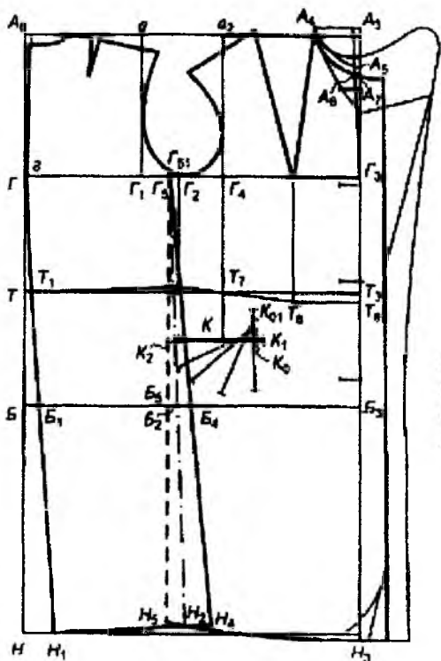
Расми 3.14. Таҳияи хатҳои паҳлӯ дар либоси тарҳи рост бо пуштаки чокдор. Таҳияи хати бари либос ва хати кеса
