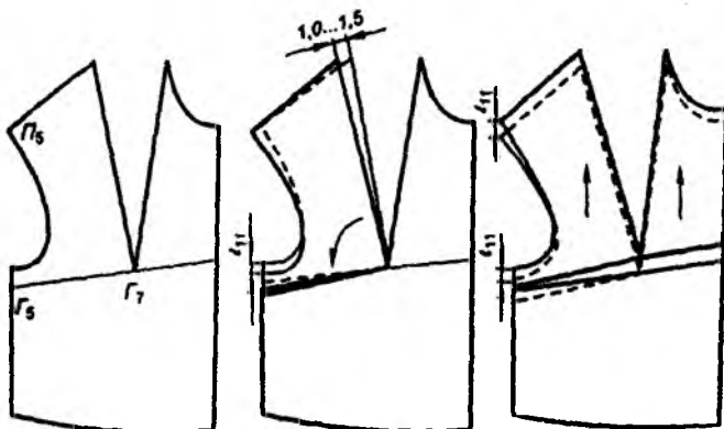
Расми 7.4. Тасҳеҳи нақшаи асоси созаи либоси китфӣ барои қомати хамида
