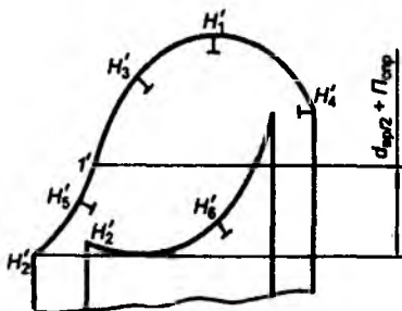
Расми 4.11. Муайянкунии мавқеи нишонаҳои (нимбурҳои) санҷишӣ дар остин ва чоки остини пиҷаки мардона, пешбар, пуштак
