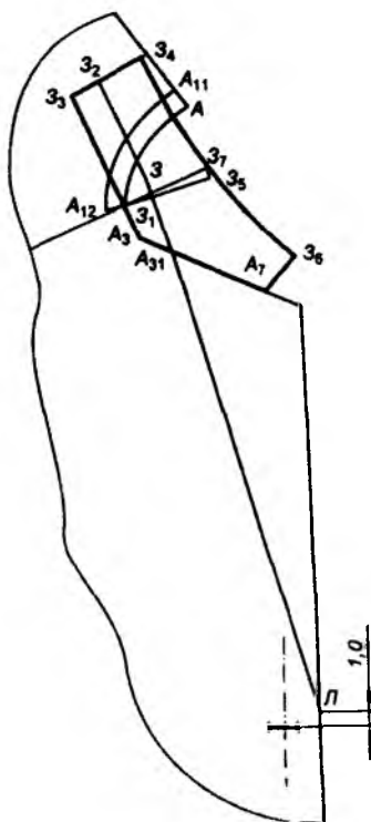
Расми 4.12. Кашидани нақшаи зергиребони пичаки мардона
