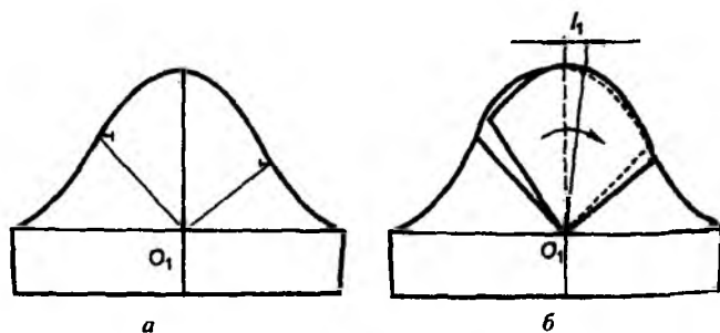
Расми 7.3. Тасҳеҳи нақшаи асоси остини даврадӯзӣ барои қомати хам
