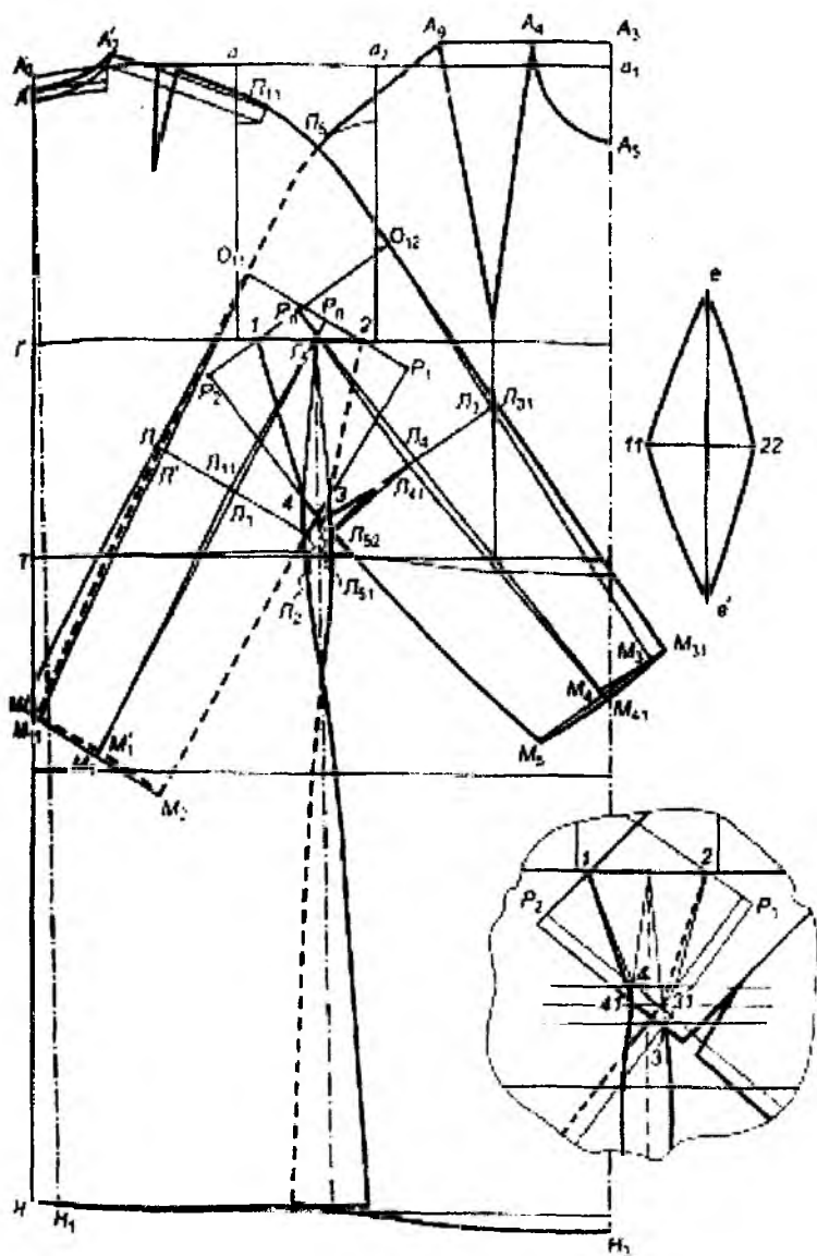
Рис. 3.38. Нақшаи либос бо остини яклухтбурида ва қуфлаки ромбшакл
