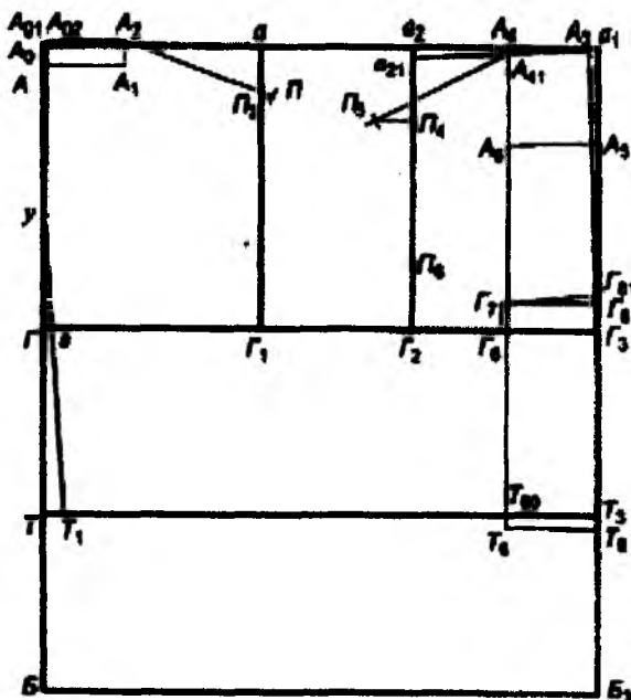
Расми 4.4. Кашидани тарҳи асосӣ ва асоси нақшаи созаи либоси китфии мардона.
