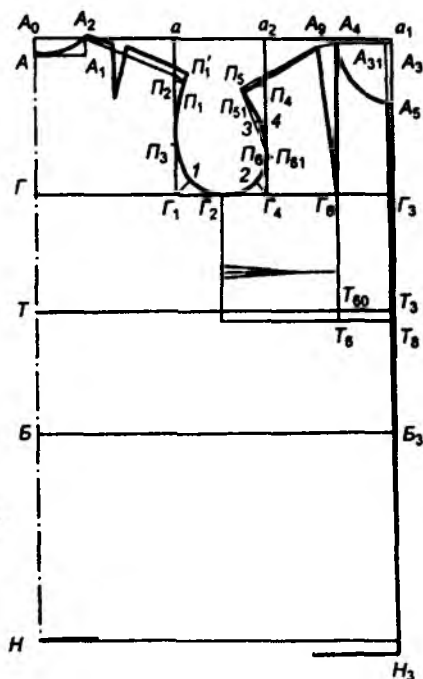
Расми 5.8. Қашдани дарзи шинам барои ҷастиди ҷистодан дар шикам дар нақшаи пешибар
