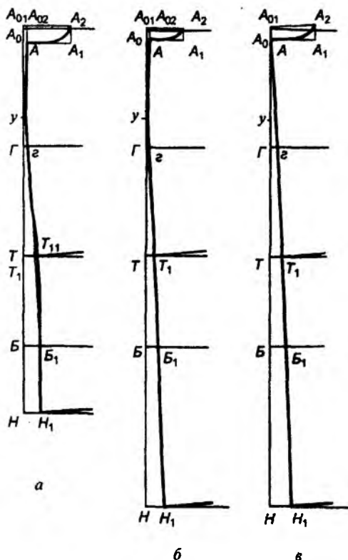
Расми 6.4. Кашидани хати мобайни пуштак
