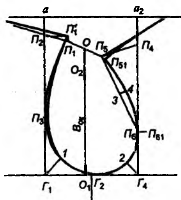
Расми 3.18. Муайянкунии баландии сари остин бо чоки сари остин дар нақшаи асоси либоси китфӣ.
