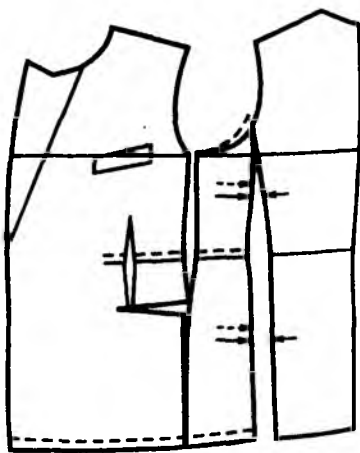
Расми 13.2. Канори пешибарҳо дар поён чудо мешаванд
