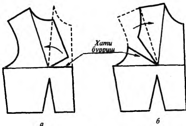
Расми 9.3. Тарзҳои ҷойивазкунии дарзи шинами пешибар (а, б)
