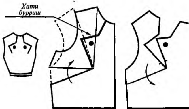
Расми 9.4. Ҷойивазкунии дарзи шинами шакли мураккаб
