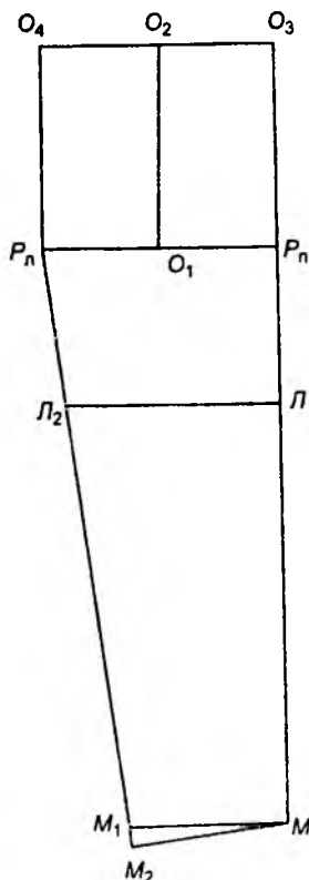
Расми 5.10. Нақшаи ҷадвал барои кашидани нақшаи асосии остини даврадӯзӣ барои духтарчаҳо
