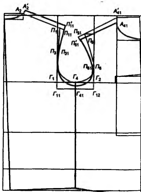
Расми 4.14. Кашидани нақшаи асоси созаи либоси китфӣ бо остини буриши куртагӣ ва чоки остини байзашакл
