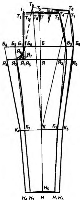
Расми 5.4. Нақшаи асоси шим барои духтарчаҳо
