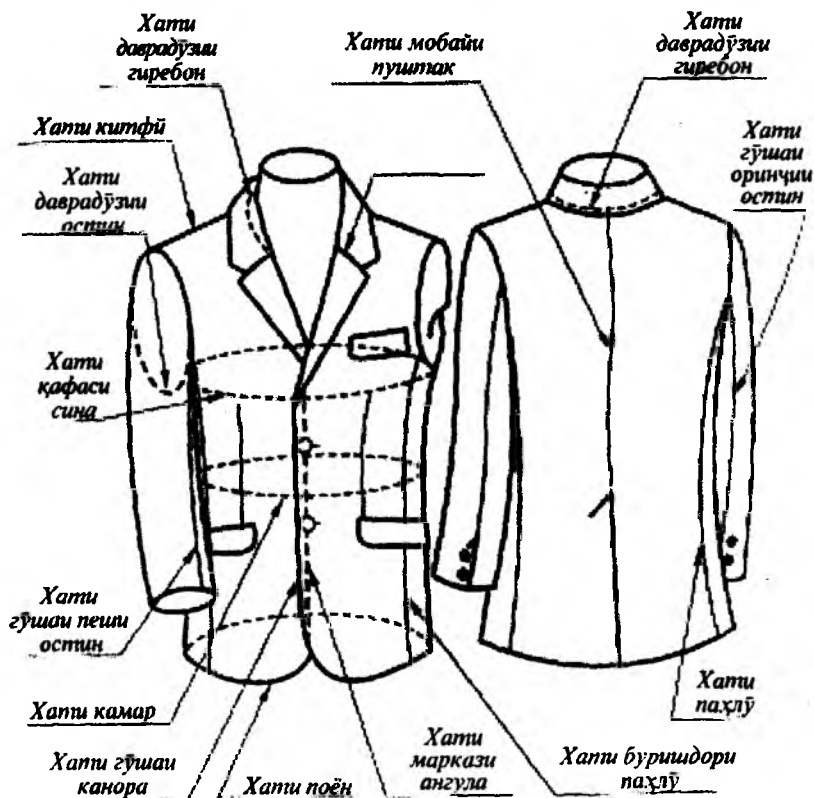
Расми 4.3. Нақшаи пичаки мардона
