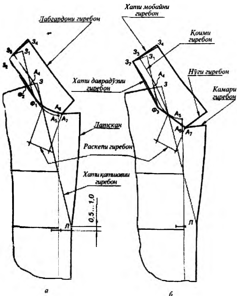
Расми 3.30. Нақшаи гиребони лабгардон барои либос бо латскан: а- дар гарданаи бийзаташкл; б- дар гарданаи мураббаъ.
