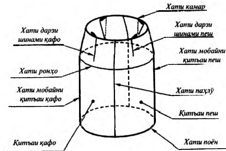
Расми 3.1. Хатҳои созаӣ ва ҷузъҳои асосии доман
