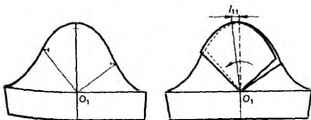
Расми 7.5. Тасҳеҳи нақшаи асоси остини даврадӯзӣ барои қомати хамида
