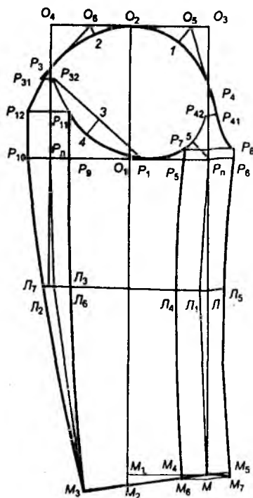
расми 6.8. Кашидани нақшаи созаи остини дучока
