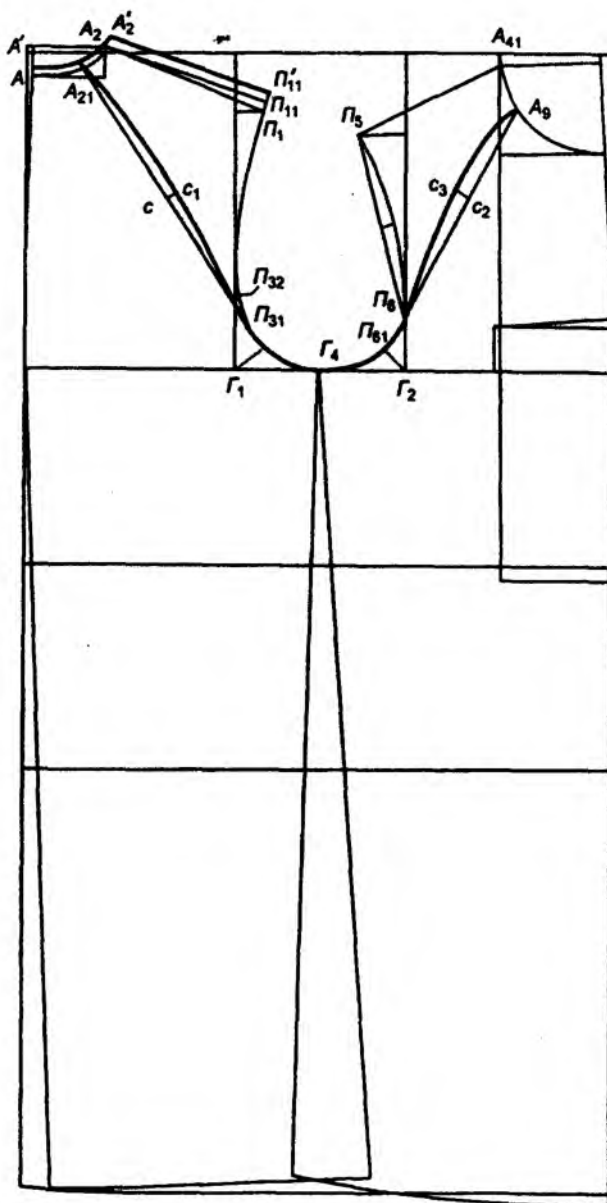
Расми 4.16. Кашидани нақшаи асоси созаи либоси китфӣ бо остини реглан ва кашидани хати реглан
