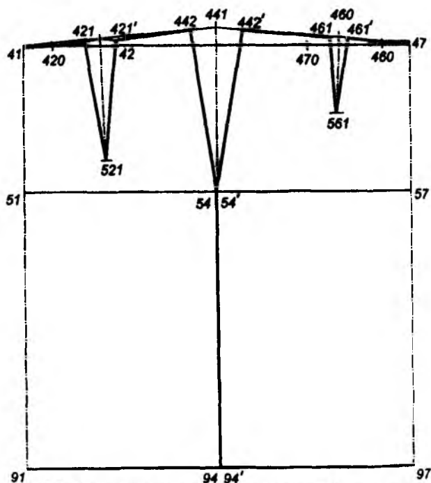
Расми 17.9. Системаи порчаҳои асосии созаии домани занона
