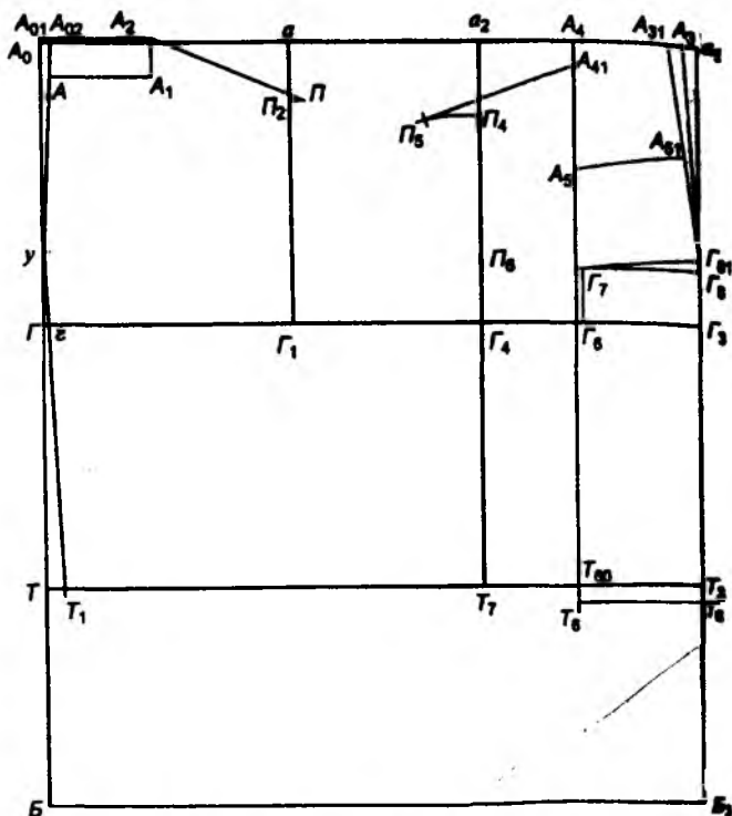
Расми 6.2 Катидани тарҳи асосии нақшаи созаи либоси китфӣ барои писарчаҳо
