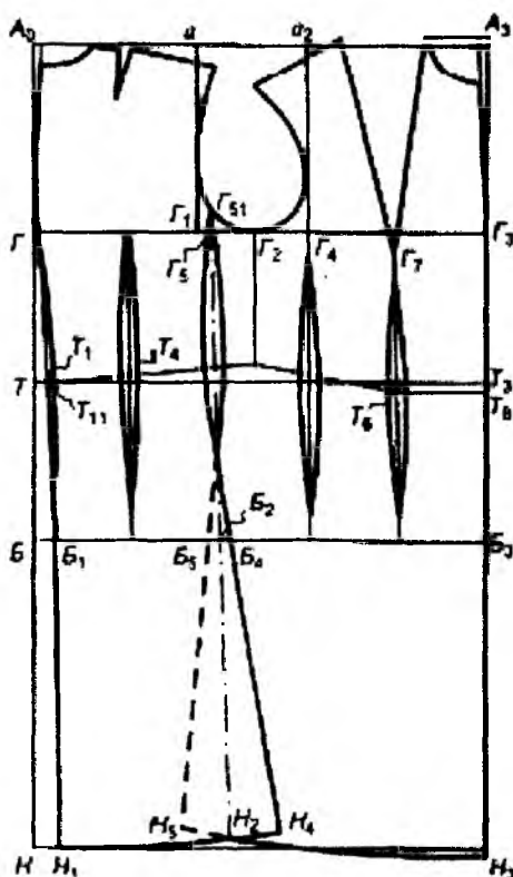
расми 3.15. Таҳияи хатҳои паҳлӯ дар либоси тарҳи нимшинам. Таҳияи хатҳои дарзҳои шинам.
