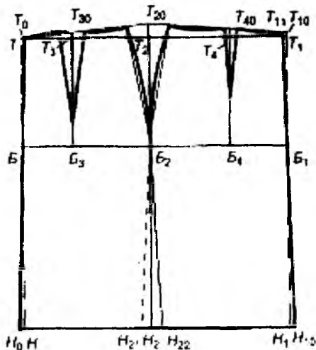
Расми 3.4. Нақшаи асоси домани рост
