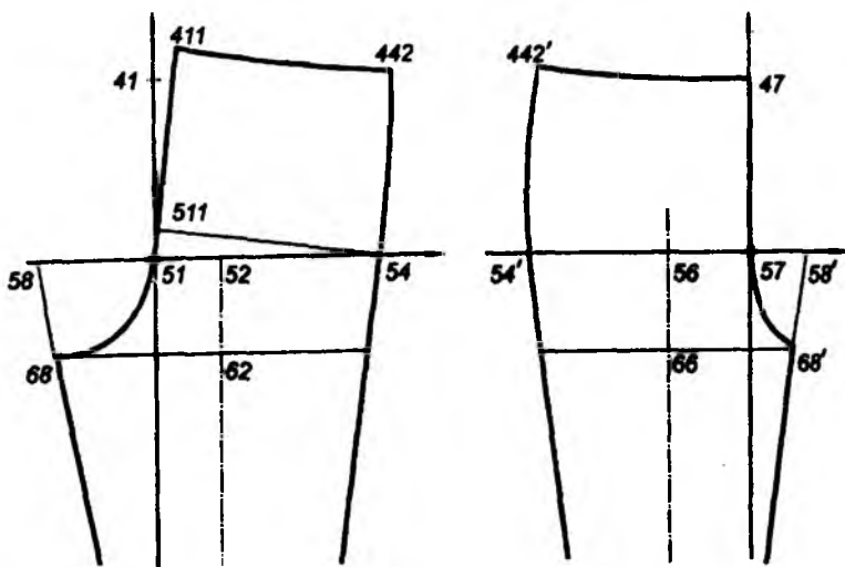
Расми 17. 8. Хатҳои ибтидоии дараҷабандӣ дар либоси камарӣ
