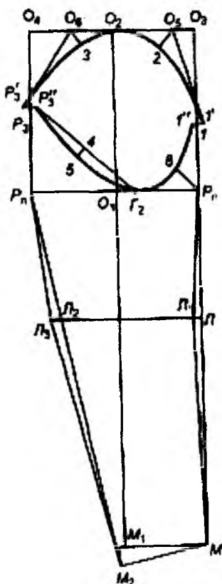
Расми 3.20. Нақшаи асоси остини даврадӯзӣ
