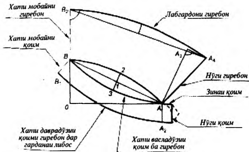
Расми 3.27. Нақшаи гиребон бо қоими буришдор.
