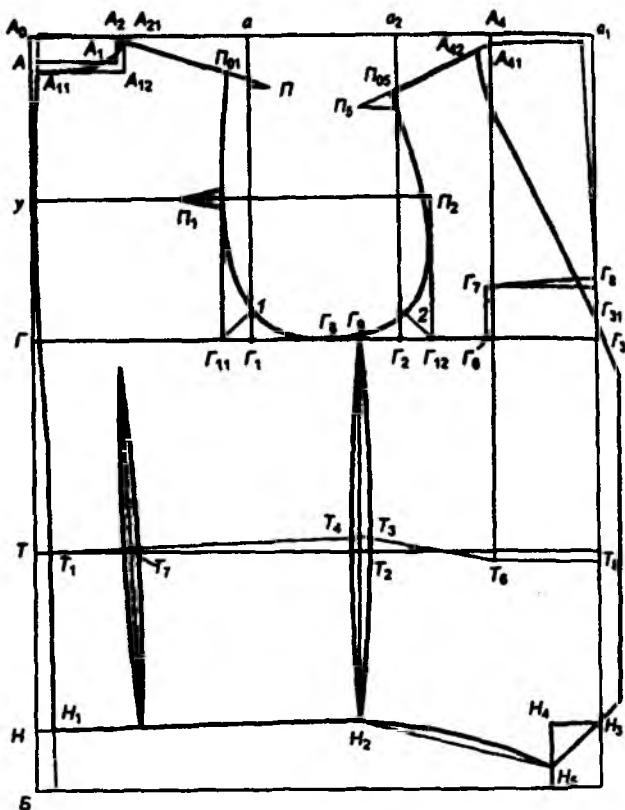
расми 4.13. Қашидани нақшаи асоси созаи нимтана.
