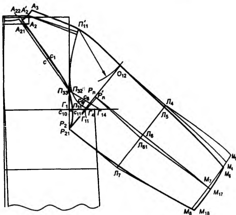
Расми 4.18. Кашидани нақшаи созаи қисми қафои остини реглан
