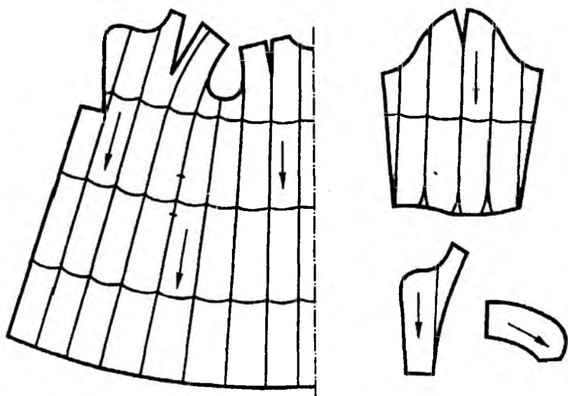
Расми 8.7. Навъи зоҳирии қолибҳои қорӣи палтои занона аз мӯинаи асли
