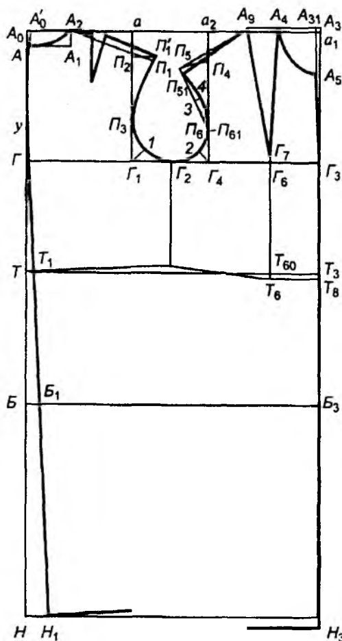
Расми 5.7. Нақшаи асоси либоси китфӣ бо остии даврадӯзӣ барои духтарчаҳо
