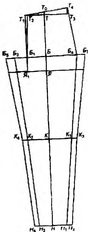
Расми 3.8. Нақшаи тарҳи асоси шими занона
