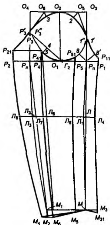
Расми 5.12. Нақшаи остини дучока барои духтарчаҳо
