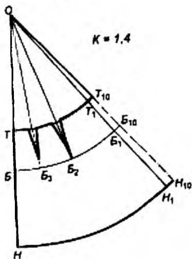
Расми 3.6. Нақшаи асоси домани махрутии васеъ
