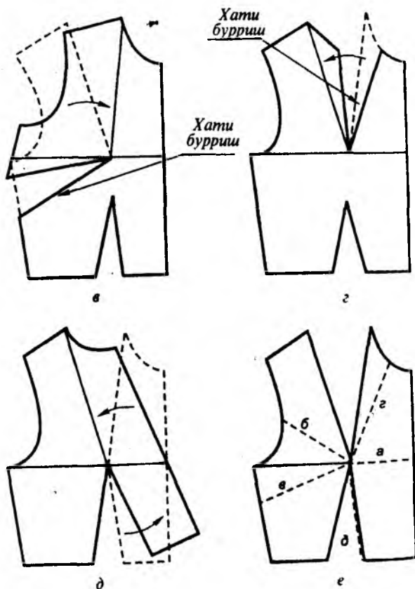
Расми 9.3. Тарзҳои ҷойивазкунии дарзи шинами пешибар (в, г, д, е.)
