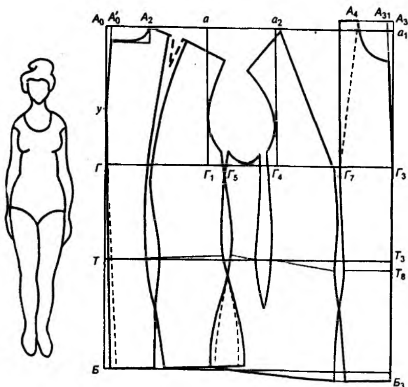
Расми 7.7. Нақшаи созаи либоси китфӣ ба ҷусса бо раванбандии зиёд дар қисми поёни бадан
