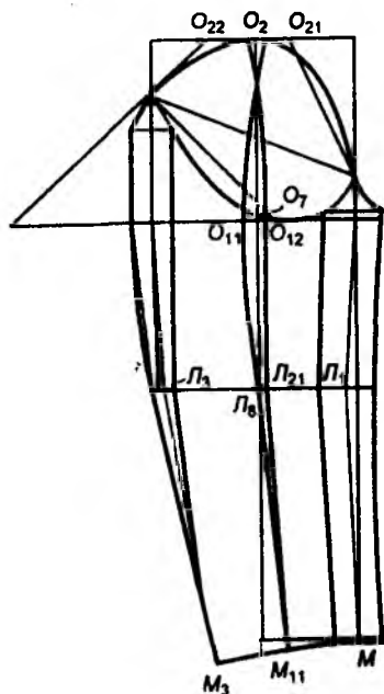
Расми 4.10. Кашидани нақшаи созаи остини сечока
