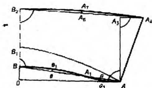
Расми 3.25. Нақшаи гиребони лабгардони ба гардан шинам
