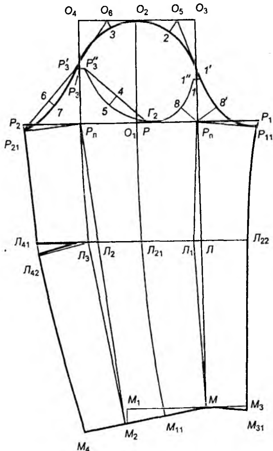
Расми 5.13. Нақшаи остини якҷока барои духтарчаҳо
