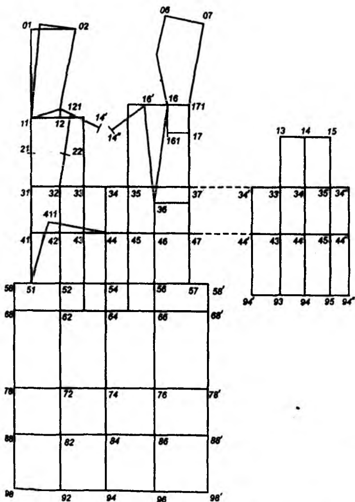
Расми 17.3. Нишонаҳои рақамии нуқтаҳои асосии созаӣ
