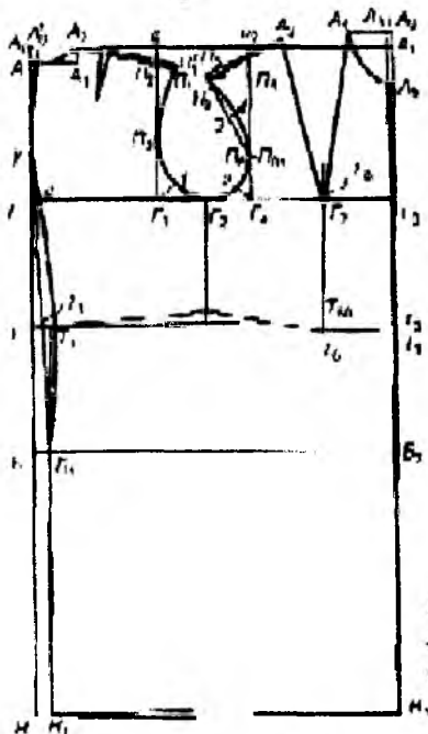
Расми 3.13. Нақшаи асоси либоси китфии занона бо остини даврадӯӣ
