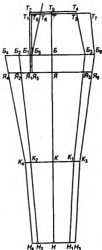
Расми 5.3. Нақшаи тарҳи асосии шим барои духтарчаҳо
