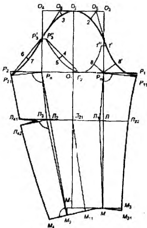
Расми 3.21. Нақшаи остини якчока
