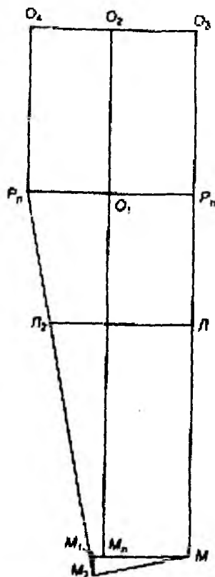
Расми 3.19. Нақшаи тарҳи асосӣ барои сохтани асоси остини даврадӯзӣ
