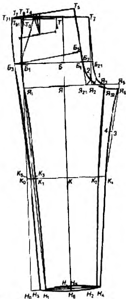
Расми 4.2. Кашидани қисмҳои пешу қафои шими мардона.
