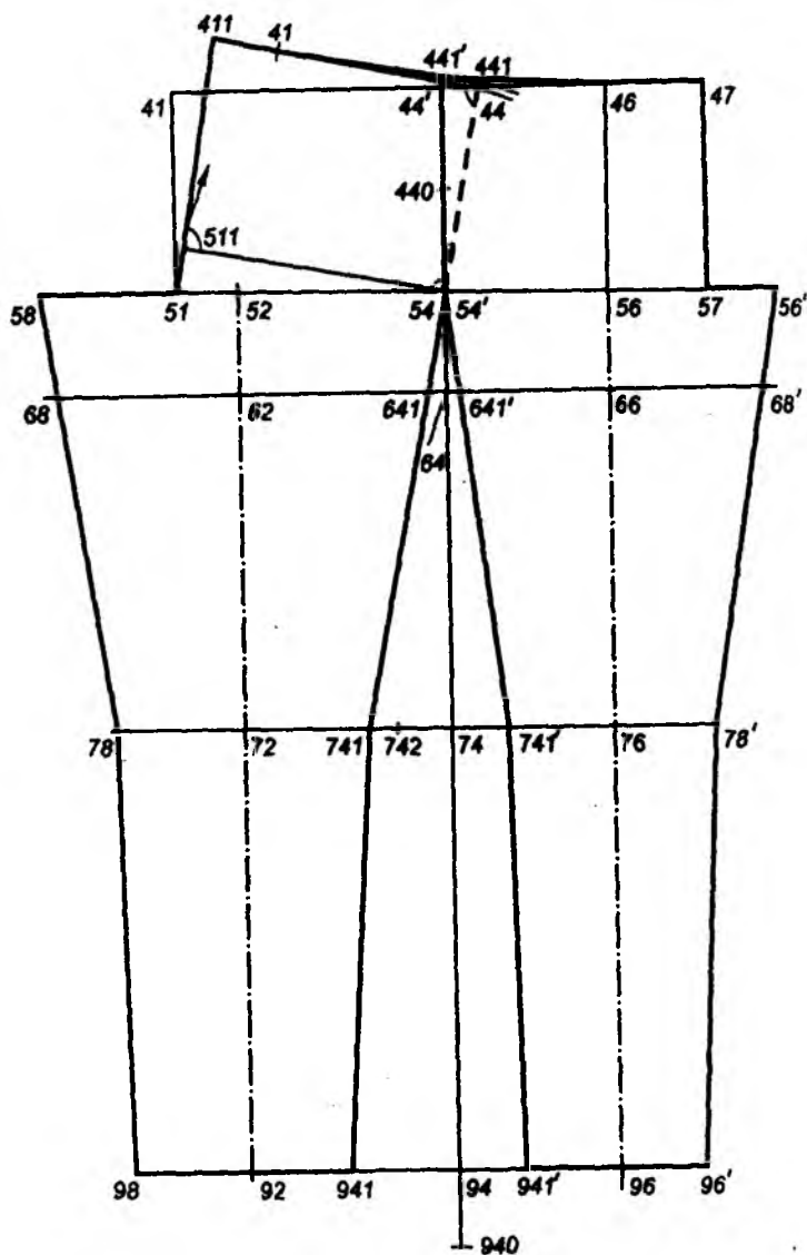
Расми 17.6. Низоми порчаҳои асосии созаии либос дар қисми поёни бадан
