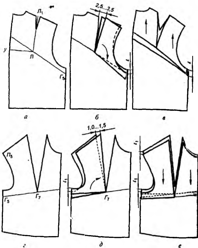
Расми 7.2. Тасҳеҳи нақшаи асоси созаи либоси китфӣ барои қомати хам
