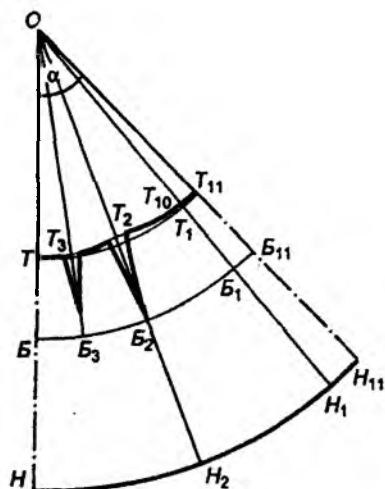
Расми 5.2. Нақшаи асоси домани махрути барои духтарчаҳо
