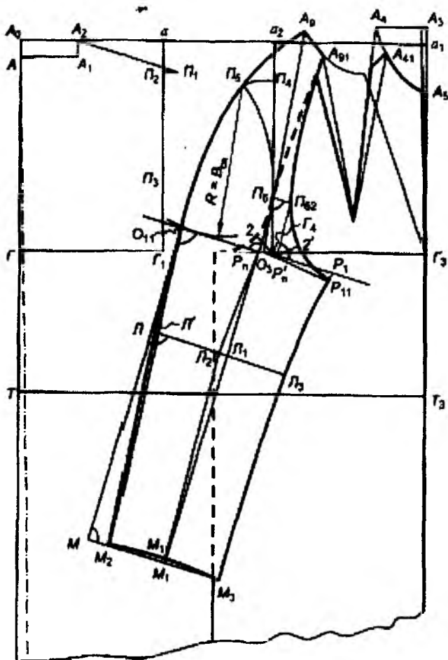
Расми 3.35 Нақшаи қисми пеши остини резлан
