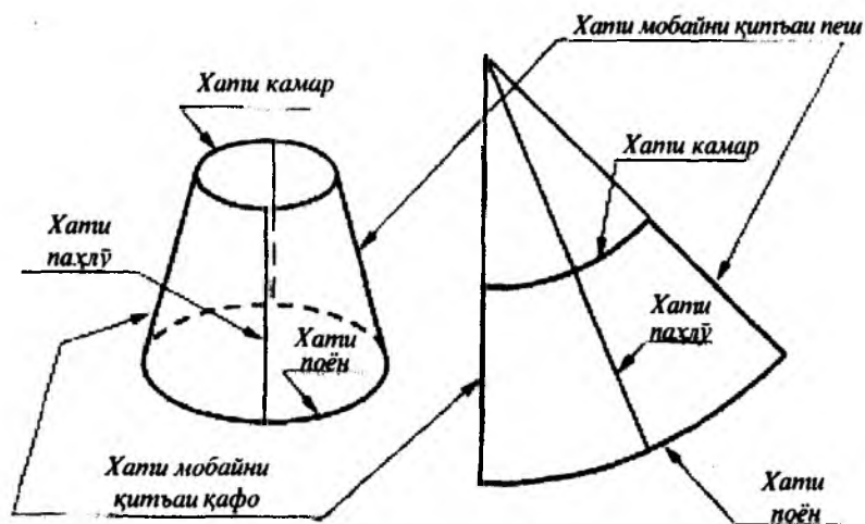
расми 3.5. Нақшаи домани махрутӣ ва густурдани чунин доман дар ҷамворӣ
