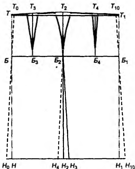
Расми 5.1. Нақшаи асоси домани рост барои духтарчаҳо
