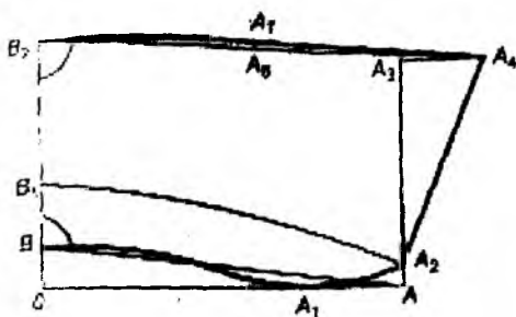
Рис. 3.26. Нақшаи гиребон бо қошқи бебуриш
