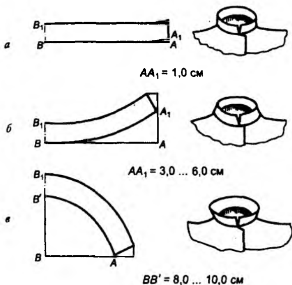
Расми 3.28. Нақшаи гиребонҳо- қоимҳо ва шаклҳои ба онҳо мувофиқи гиребонҳои тайёр.
