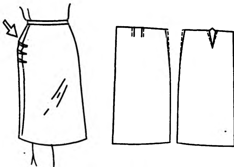
Расми 13.15. Сустӣ бо чоки паҳлӯ дар қисмати ронҳо
