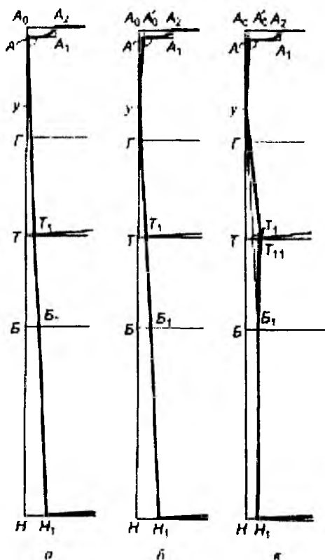
Расми 3.12. Кашидани хати мобайни пуштаки либоси китфии занона.
