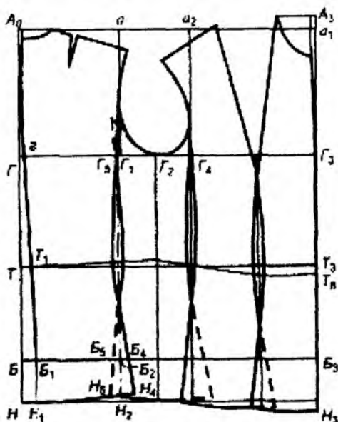
Расми 3.16. Таҳияи хатҳои паҳлӯ дар либоси тити пичак. Таҳияи хатҳои муқарнас.
