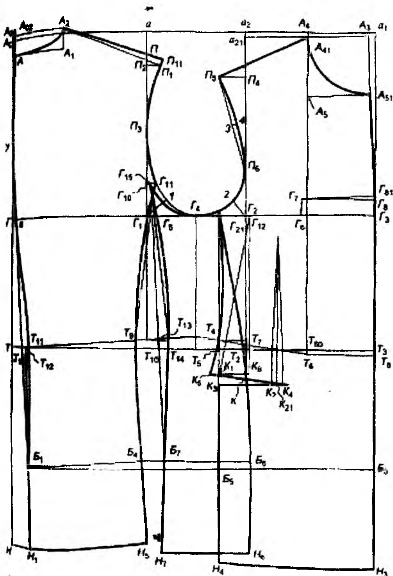
Рис. 4.6 Кашидани нақшаи сози пиҷаки мардона
