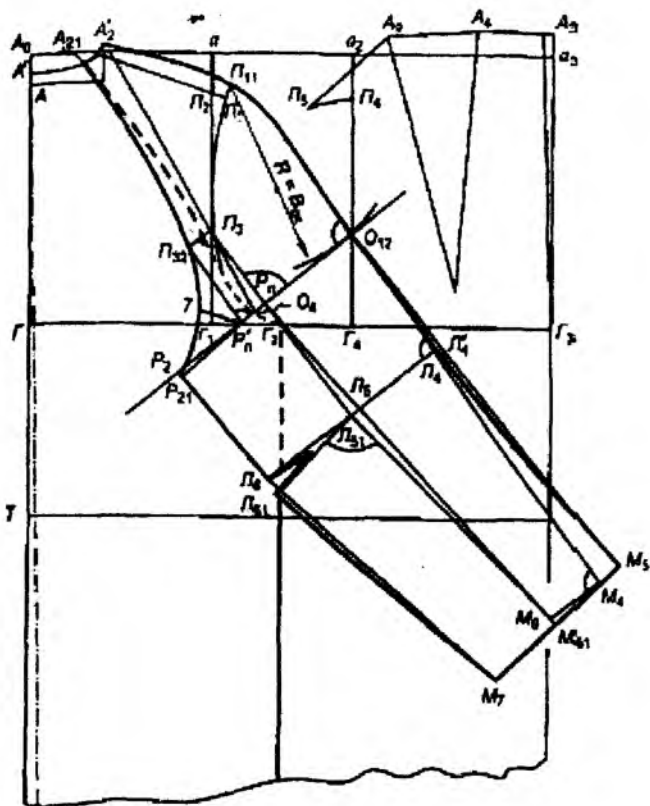
Расми 3.36. Нақшаи қисми қафои остини реглан
