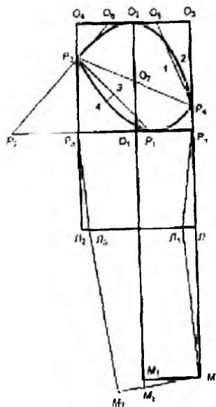
Рисми 4.7. Кашидани тарҳи асосӣ ва нақшаи асоси остини давридузӣ
