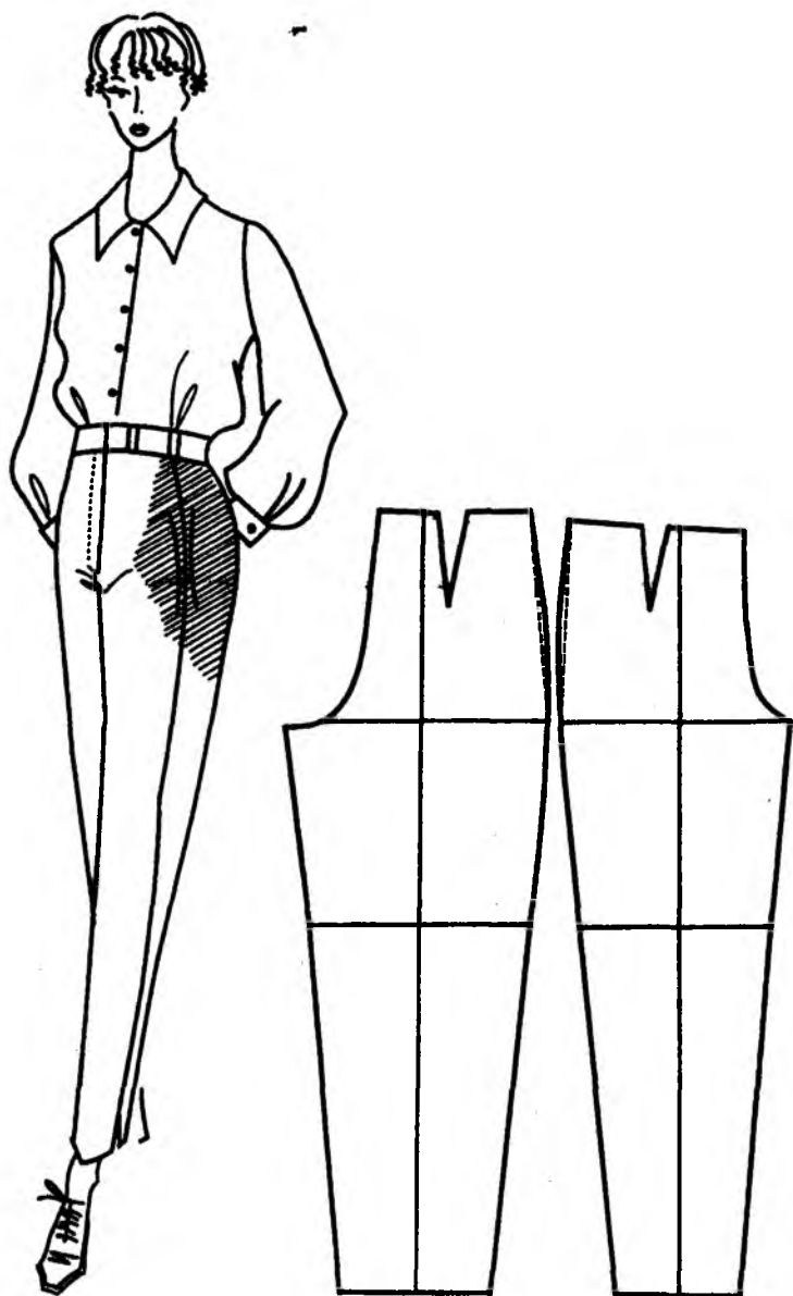
Расми 13.19. Чини амудӣ дар нимаҳои қафо қад-қади чоки пахлӯ дар қисмати ронҳо
