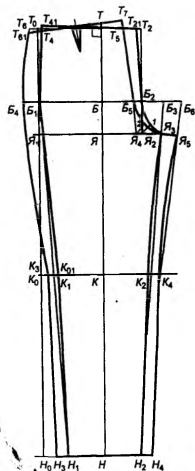
Расми 6.2. Кашидани қисмҳои пешу қасрои шим барои писарчаҳо
