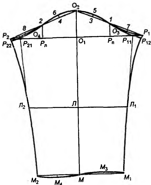
Расми 4.15. Кашидани нақшаи созаи остини буриши куртагӣ
