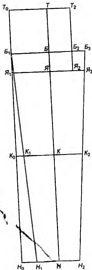
Рис. 6.2. Қашидани қисмҳои пешу қафои шим барои писарчаҳо
