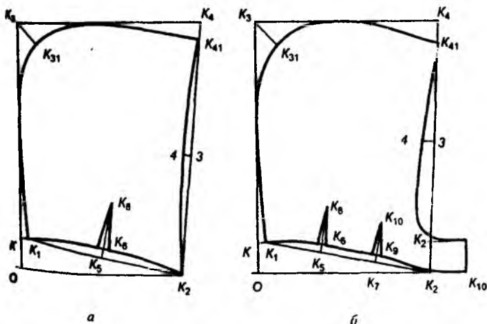
Расми 6.11. Нақшаи созаи капюшонҳо
