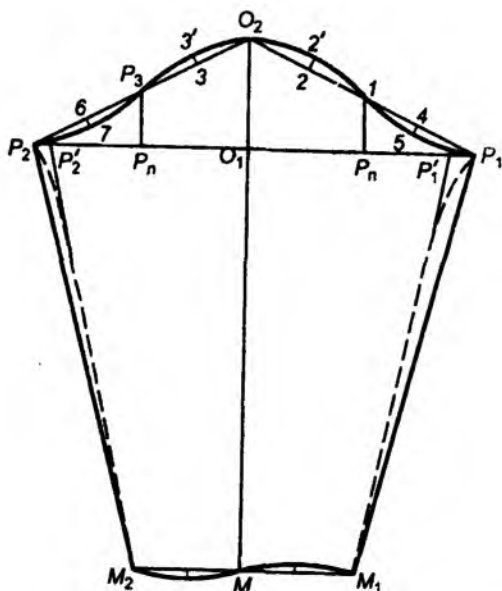
Расми 3.33. Нақшаи остини буриши куртағӣ.
