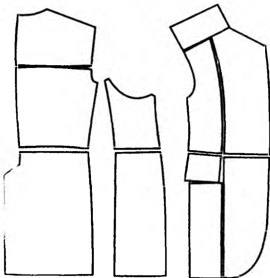
Расми 8.1. Намунаи ҷудокунии ҷузъҳои асосии пичаки мардона аз чармӣ аслӣ
