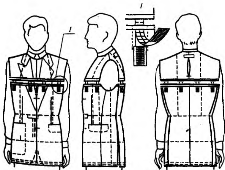
Расми 16.2. Созаи нимтанаи универсалии андозавӣ
